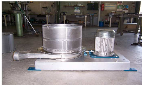
Centrifugadora de granza
