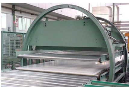
Sistema de transporte y volteado a 180°
