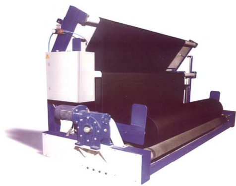
Enrolladora de tejido
