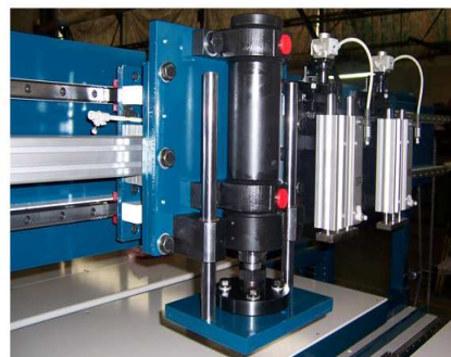
Automatisation combiné hydraulique et pneumatique
